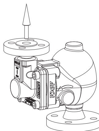
VT - Вертикальний вхідний та вихідний патрубки, напрямок потоку знизу вгору
