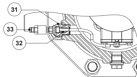
FLL - Важіль підйому поплавка
