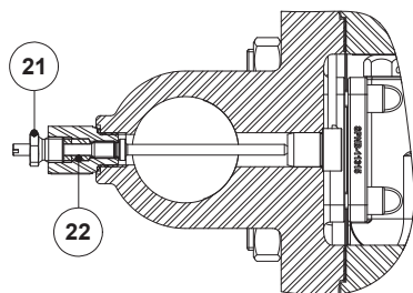
SLR - Клапан для випуску парових пробок
