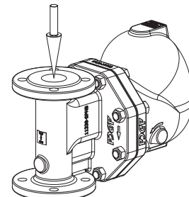
Встановлення на вертикальному трубопроводі, напрямок потоку зверху вниз (IT).
