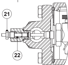
SLR - Клапан для випуску парових пробок
