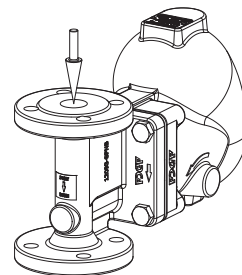
Встановлення на вертикальному трубопроводі, напрямок потоку зверху вниз (IT).
