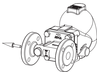
Встановлення на горизонтальному трубопроводі, напрямок потоку справа наліво (IR).
