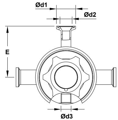
Приєднання для манометра
