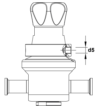
Додаткове з'єднання для вентиляції газів та/або витоку робочого середовища
