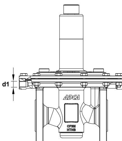
Лінія відбору імпульсу тиску за клапаном
