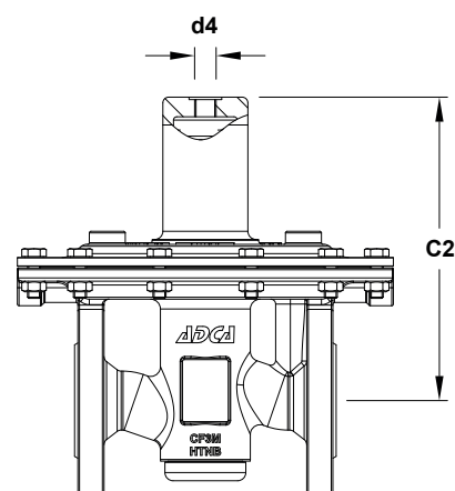
Купольна кришка з пілотним керуванням (опція)
