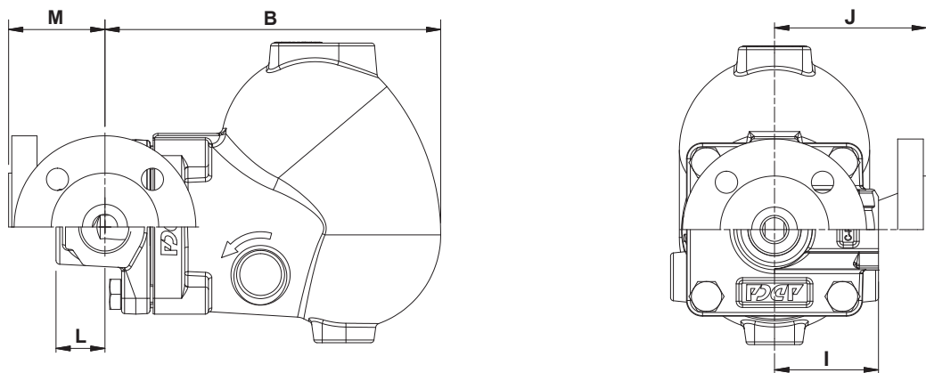
Кутова конструкція
