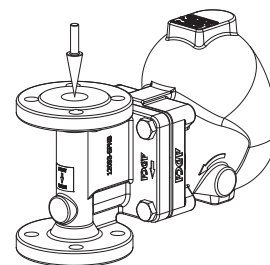
Встановлення на вертикальному трубопроводі, напрямок потоку зверху вниз (IT).
