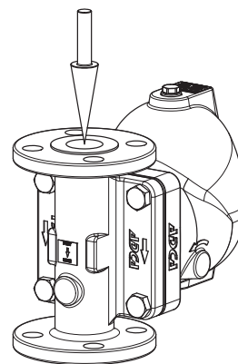
Встановлення на вертикальному трубопроводі, напрямок потоку зверху вниз (IT).
